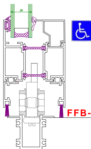
Straßencafeschwelle
