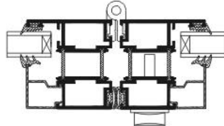
Autohausschwelle
