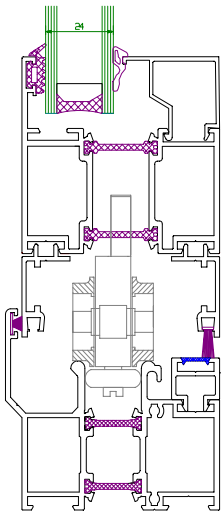
Normalausführung
